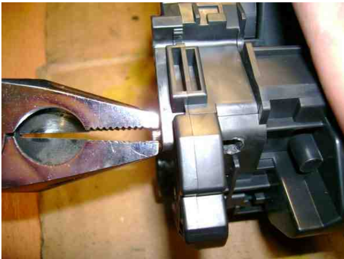
5. Разделяем картридж на две половины.
